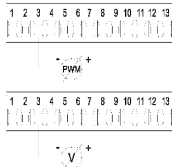
Εικόνα 8: Αφαιρούμενη κλέμμη 13 πόλων: είσοδος 0-10V και PWM
