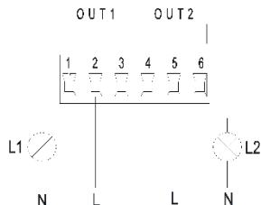
Figura 9: Morsettera estraibile 6 poli: esempio di collegamento uscite
