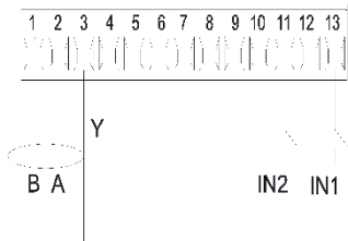
Attēls 7: Izņemams spaļu panelis ar 13 kontaktiem: digitālās ieejas un
