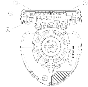
5. ábra: elektromos bekötések (háttoldal)
