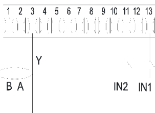
Rys. 7: Skrzynka zaciskowa na 13 biegunów: cyfrowe wejścia i MODBUS
