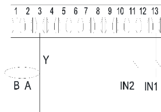
Obr. 7: Vyjimatelná 13 pólová svorkovnice: digitální vstupy a MODBUS
