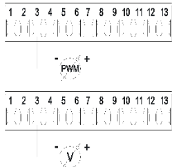
Figura 8: Barra de terminais extraível 13 pólos: Entradas 0-10V e PWM
