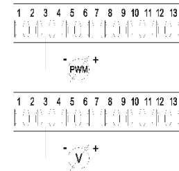
Obr. 8: Vyberateľná 13-pólová svorkovnica: vstupy 0-10V a PWM
