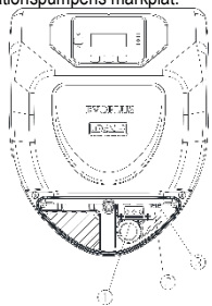
Fig. 4: Elanslutning (framsida)
