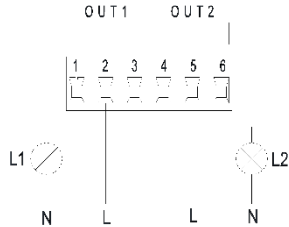
Obr. 9: Výměnitelná 6 pólová svorkovnice: příklad připojení výstupů
