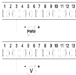
Abbildung 8: Abnehmbares Klemmbrett mit 13 Polen: Eingänge 0-10V und PWM
