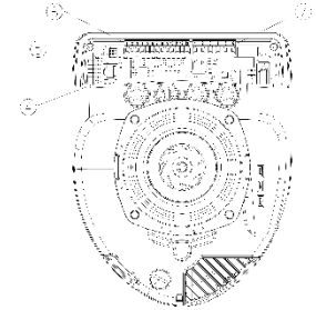
Εικόνα 5: Ηλεκτρική συνδεσμολογία (πίσω μέρος)
