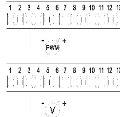
8 pav. Ištraukiama 13 kontaktų gnybtų dėžutė. Įvadai 0-10V ir PWM
