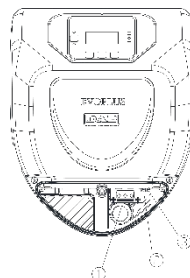
Figura 4: Connessioni elettriche (fronte)
