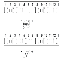
Figure 8 : Bornier amovible 13 pôles : entrées 0-10V et PWM
