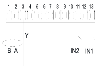
Figura 7: Morsetteria estraeibile 13 poli: ingressi digitali e MODBUS
