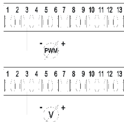
Figura 8: Morsettera estraibile 13 poli: ingressi 0-10V e PWM
