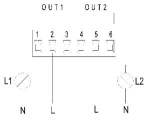
Εικόνα 9: Αφαιρούμενη κλέμμη 6 πόλων: παράδειγμα σύνδεσης εξόδων
