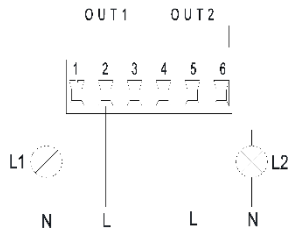
Abbildung 9: Abnehmbares Klemmbrett mit 6 Polen: Beispiel für den Anschluss der Ausgänge
